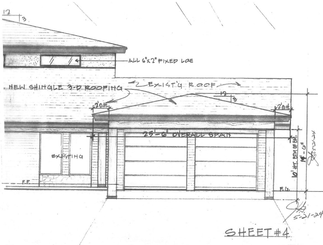
ELEVATION 2
