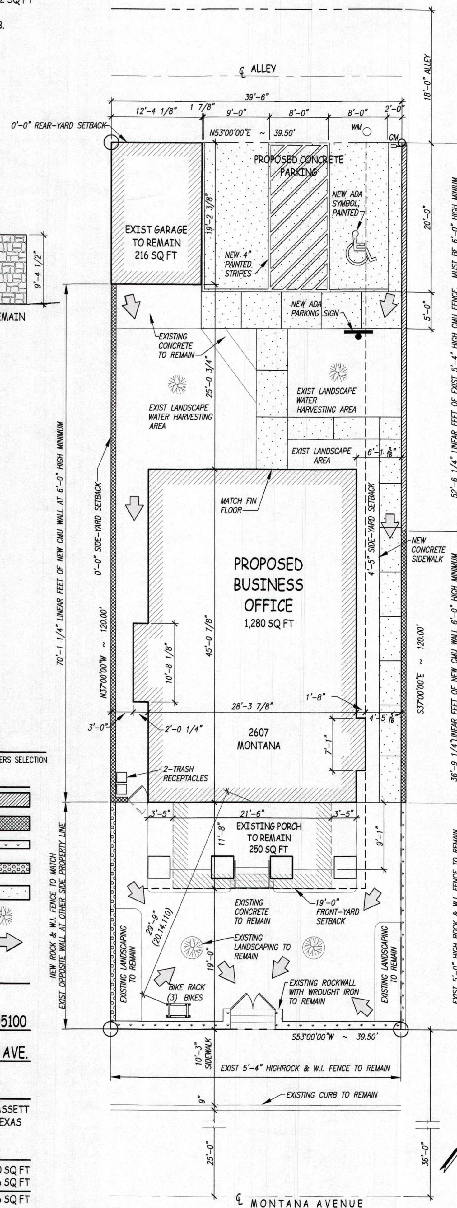
A4 SITE PLAN 1/8"=1'-0"
